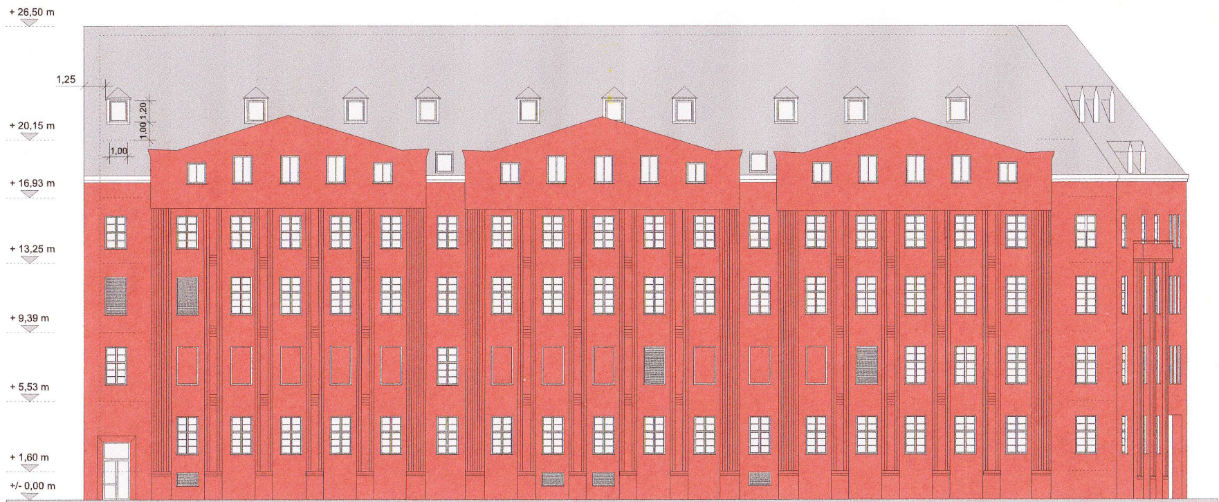
Straßenansicht Juliusstraße
